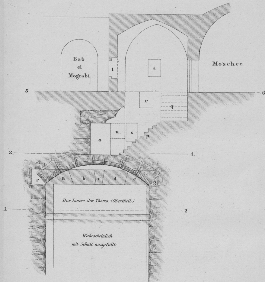
Durchschnitt II nach der Linie CD der Grundrissse.
