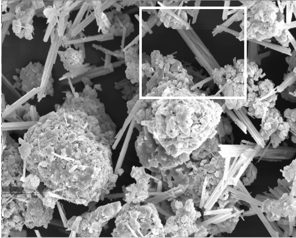
Abb. 29: REM-Aufnahme der hydratisierten Abmischung P30; Ettringit und unhydratisierte Phase; Bildbreite = 67 \mu\text{m}
