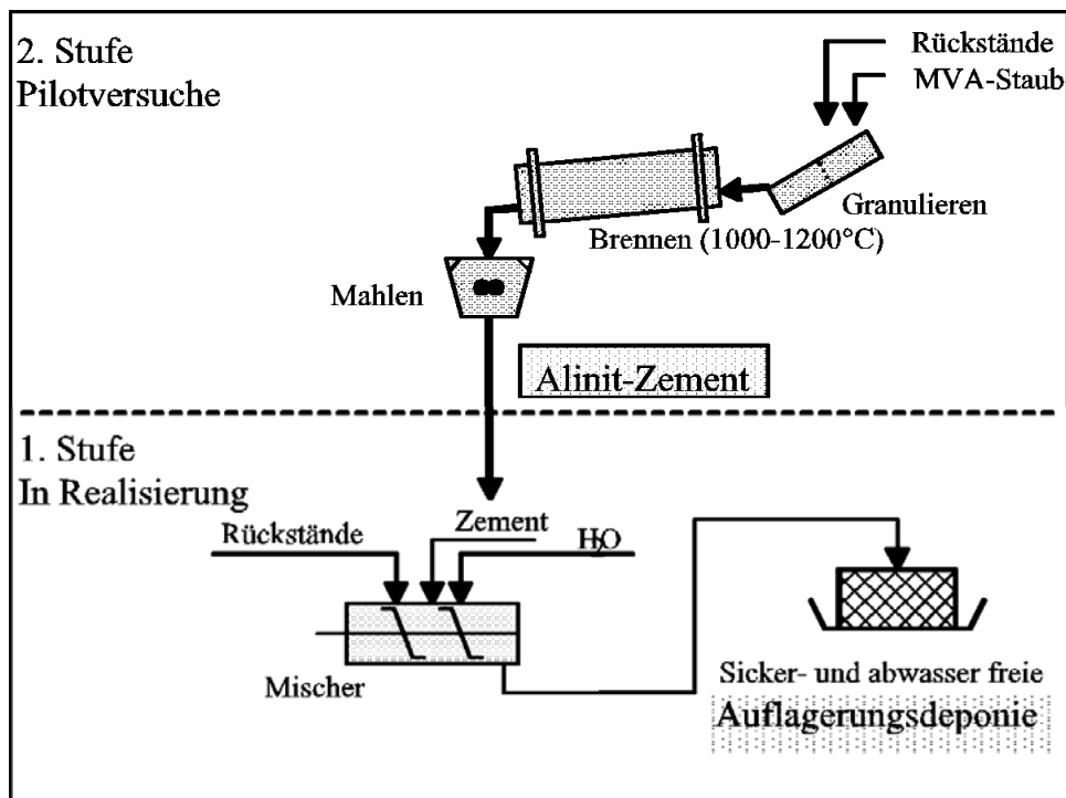
Abb. 34: Zweistufiges Konzept einer Auflagerungsdeponie nach RHEINISCHE KALKSTEINWERKE GmbH (Wülfrath) (1992)
