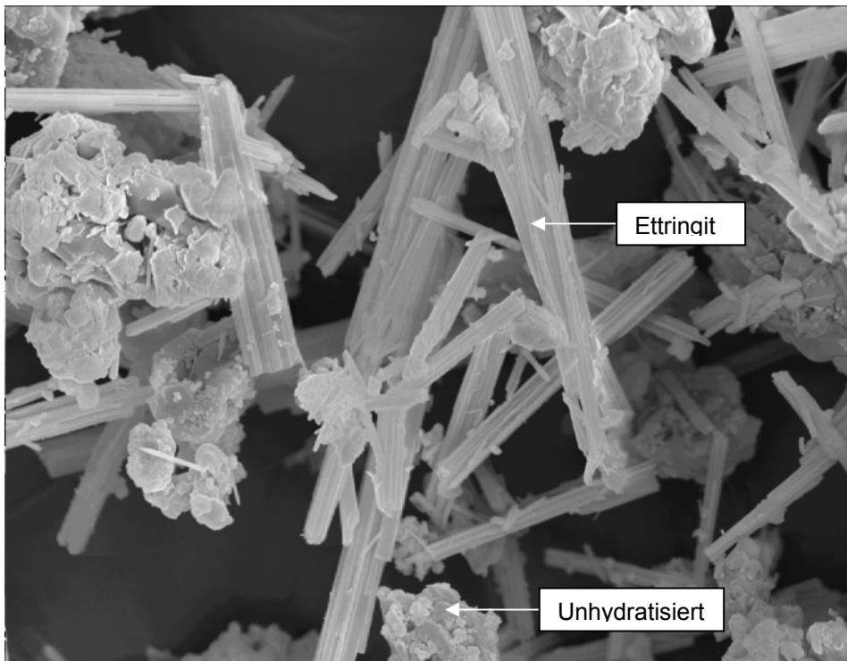
Abb. 30: REM-Aufnahme der Ausschnittsvergrößerung von Abb. 28 der Abmischung P30; Ettringit und unhydratisierte Phase; Bildbreite = 67 \mu\text{m}
