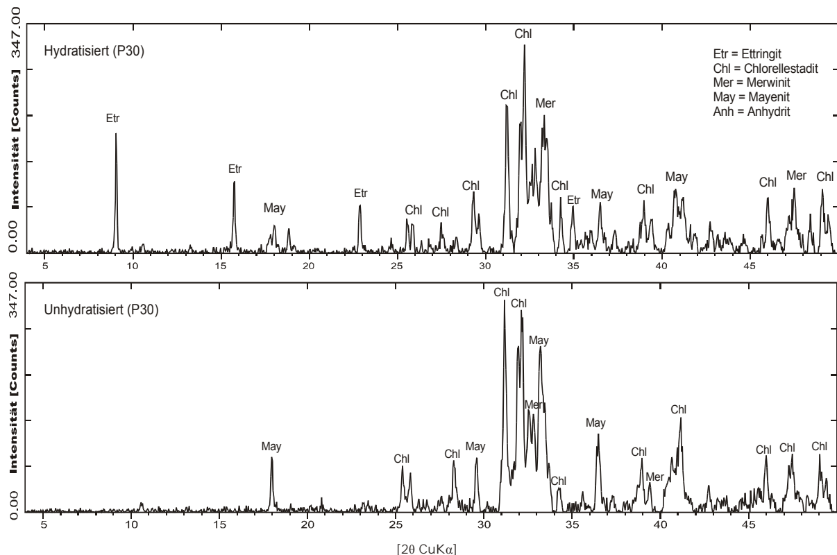
Abb. 27: Die mineralogischen Phasen der thermisch (halbtechnischer Versuch im Drehrohrföfen bei 1000^{\circ}\text{C}/25 Minuten - unteres Diagramm) und die zusätzlich zur thermischen Behandlung auch hydraulisch (Hydratationszeit von 24 Stunden – oberes Diagramm) behandelten Abmischung P30
