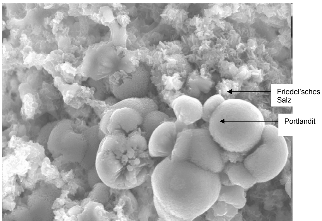
Abb. 41: REM-Aufnahme der hydratisierten Abmischung B19; Bildbreite = 57\mu\text{m}
