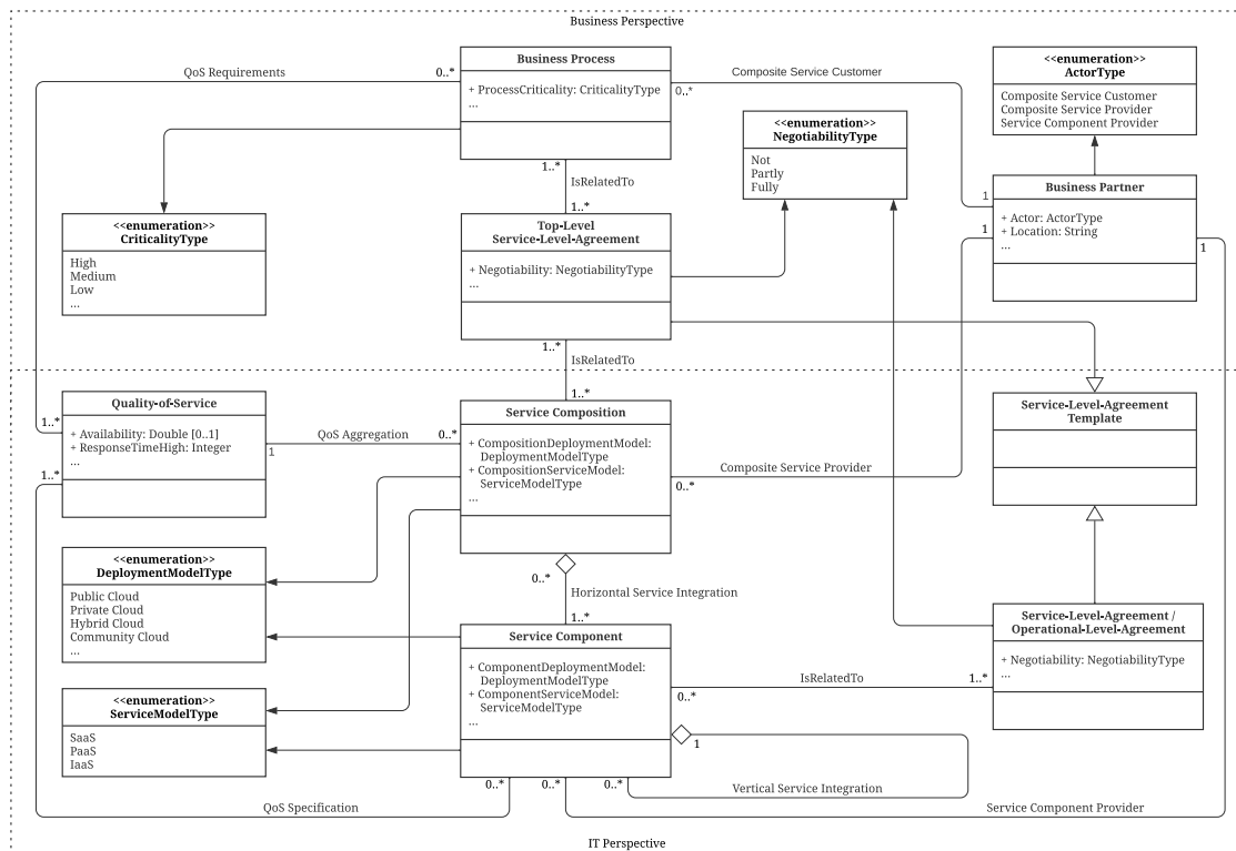
Das konzeptuelle HySLAC-Modell als Klassendiagramm in UML 2.0
