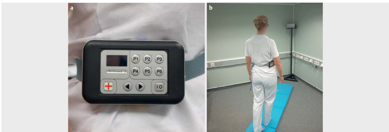
► Abb. 4 Beispiel für ein Oberkörperschwankungs-Messsystem: Vertiguard (Zeisberg, Metzingen, Germany) welches an der Hüfte in der Nähe des Körperschwerpunktes getragen ( a ) mittels Beschleunigungssensoren die Oberkörperschwankung erfasst. b: Einsatz zur dynamisch-mobilen Messung beim Gehen auf Schaumstoffmatten mit frontaler Schallpräsentation in echoarmer Kabine.
