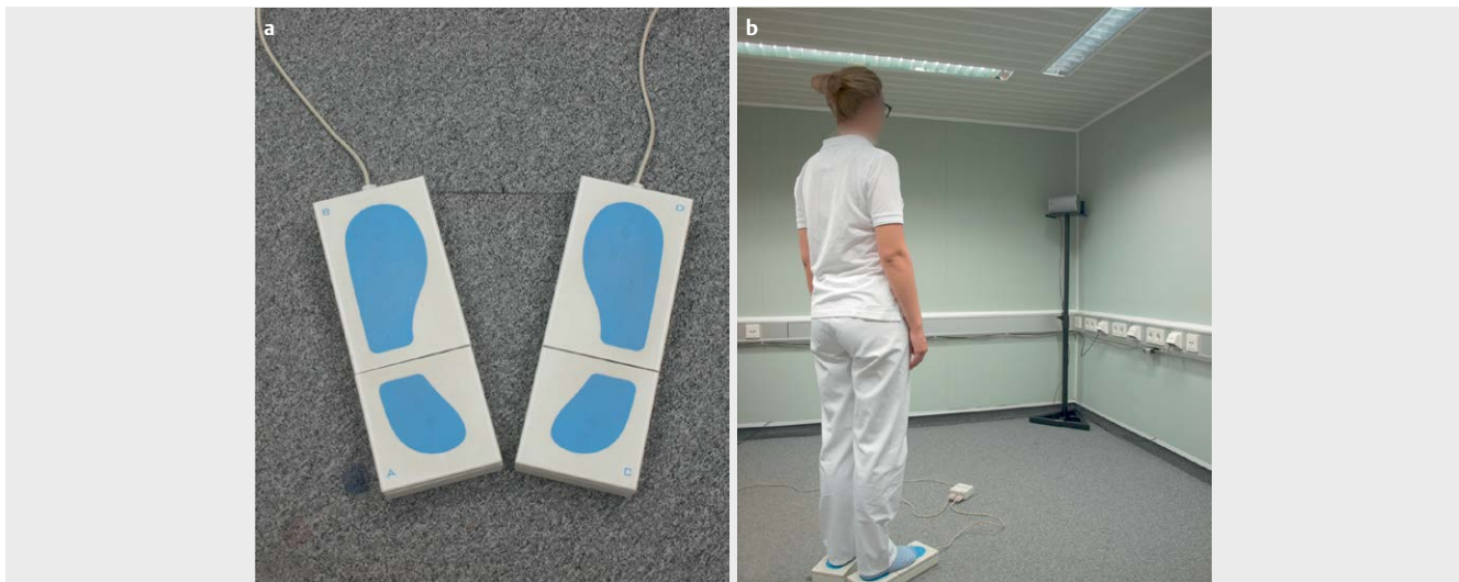
► Abb. 3 Beispiel für ein Fußplatten-Messsystem: IBS, (IBS Interactive Balance System (Fa. neurodata GmbH, Wien, Österreich), welches zusätzlich zu Kräfteschwankungen zwischen Vor- und Rückfuß mittels frequenzorientierter Fast-Fourier-Analyse des Kraft-Zeit-Signals eine Analyse posturaler Subsysteme ermöglicht [104, 105] a: Fußplatten, angeordnet im 30° Winkel b: Einsatz bei Messung mit frontaler Schallpräsentation in echoarmer Kabine.
