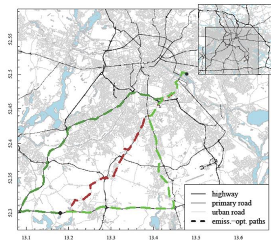
Emissionsminimale Wege von einem Warenverteilzentrum in die Innenstadt von Berlin in Abhängigkeit vom Fahrzeugtyp, der Tageszeit und dem Beladungszustand
