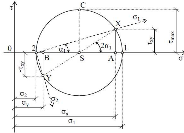
Fig. 82 – Mohr circle
