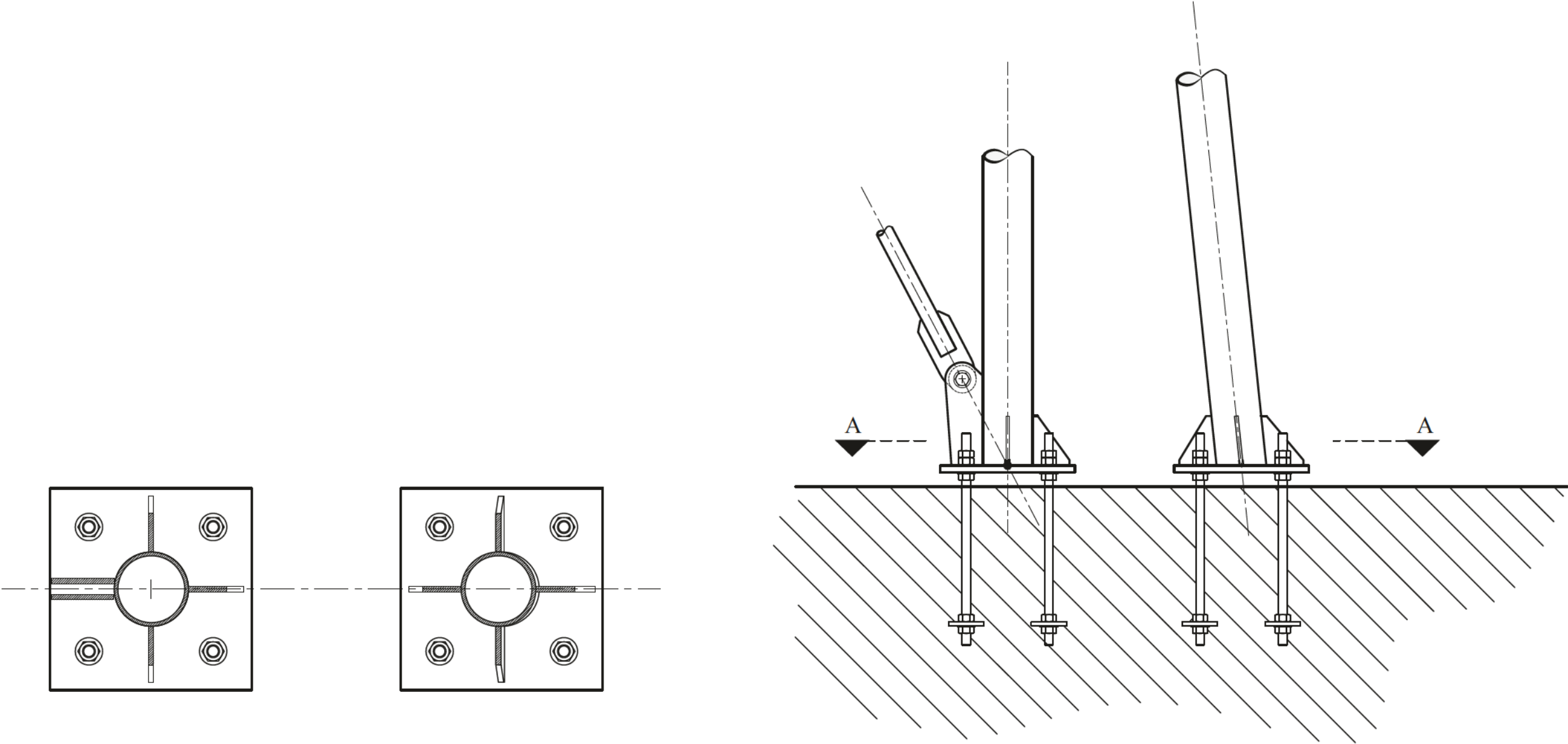
Section A-A
