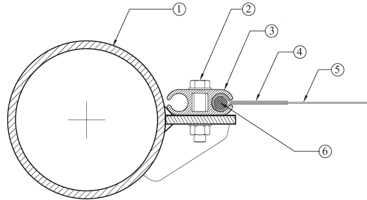
Section A-A
