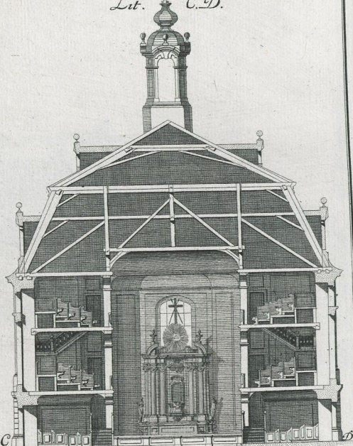
Profil durch die Garnisons Kirche. Lit. C. D.
