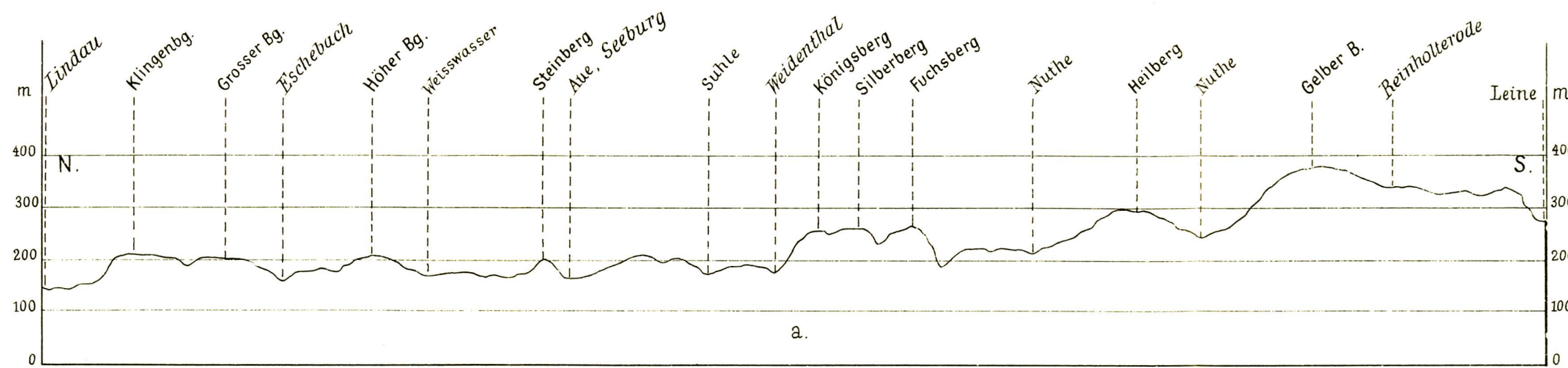
I. Längsprofil durch das Eichsfeld von Lindau bis Katharinenberg (55,6 Kilometer.) a) Lindau - Leine (29,45 Kilometer.)
