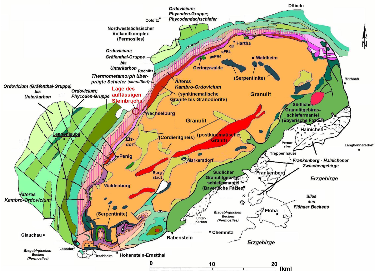
Abb. 7 Schematische geologische Übersichtskarte des Sächsischen Granulitgebirges. Senkrecht schraffiert: Garben- und Fruchtschiefer in der nördlichen inneren Schieferhülle; Garbenschiefer kommen zwischen Penig, Wechselburg und Rochlitz vor. Lage des ehem. Garbenschiefer-Steinbruchs, der mutmaßliche Herkunftsort der Platte des Melanchthon-Tischs..
