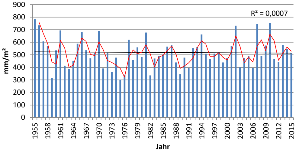
Abb. 21 Niederschlag (unkorrigiert) (Jahr) von Magdeburg in mm/m 2 mit gleitendem Mittel und Trendgerade ( R^2 = Bestimmtheitsmaß).
