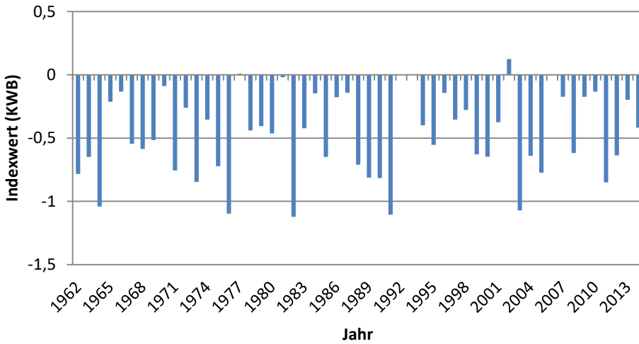
Abb. 3 Klimatische Wasserbilanz (KWB) (Jahr) von Artern.
