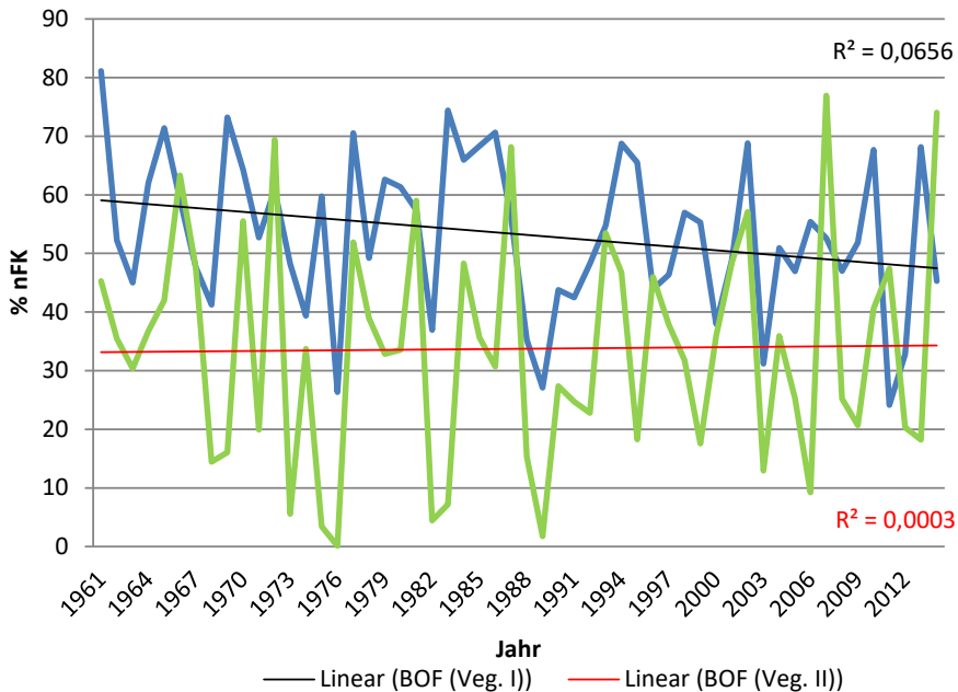
Abb. 20 Bodenfeuchte (Vegetationsperioden) von Magdeburg in Prozent der nutzbaren Feldkapazität (% nFK) (blaue Linie: Vegetationsperiode I; grüne Linie: Vegetationsperiode II) mit Trendgeraden ( R^2 = Bestimmtheitsmaß).
