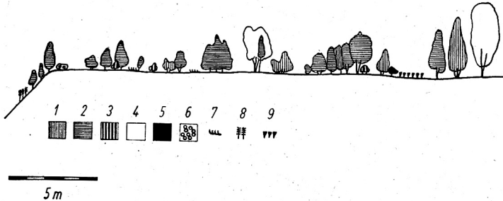
Abb. 6. Vegetationsprofil durch eine Wismuthalde bei Neustädtel. Haldengestein: blättrig verwitterter Gneis. Profilbreite etwa 2 m. Bei normal entwickelter Haldenvegetation bedecken in der Pioniergesellschaft Birken zu ungefähr 50 % die Fläche. Schnitt: NNE-SSW. Sept. 62
