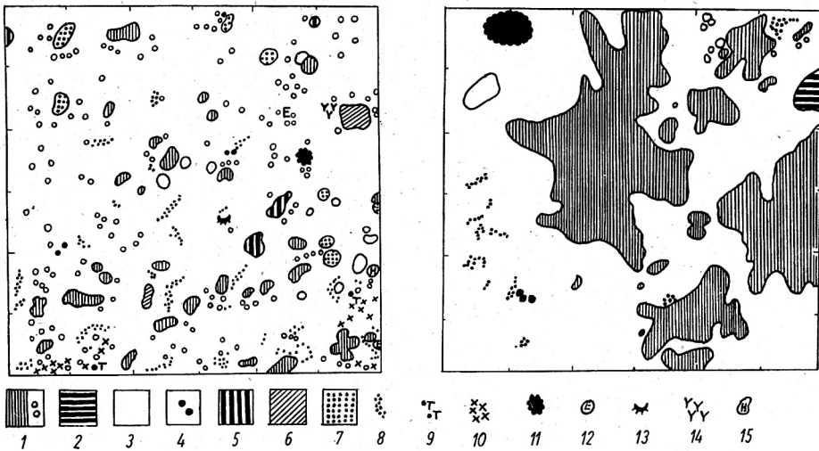
Abb. 10. Deckungsverhältnisse in der Pioniergesellschaft. Links: zweijähriges Entwicklungsstadium auf dem Konstantinschacht bei Zug; rechts: zwölfjähriges Stadium, Frohnau. Fläche je 12 \times 12 dm.
