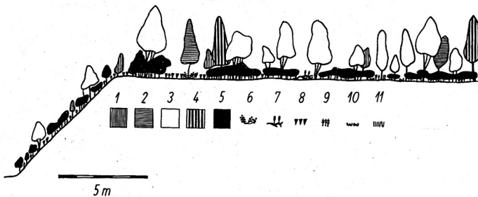
Abb. 8. Standorte wie bei Abb. 7. Auf dem grusigen Granitzersatz entwickelte sich eine ausgesprochene Picea abies -Variante der Pioniergesellschaft mit optimal entwickelter Kiefer, einer reichen Kryptogamenflora, ( Cladonia chlorophaea , — cornutoradiata — glauca , — coniocraea , — fimbriata , — gracilis , — cornuta , — furcata , — deformis , — macilenta , — bacillaris und die sehr seltene — impexa ; wichtig ist das Vorkommen von mehreren autochthonen, bis 60 cm langen Sprossen von Lycopodium clavatum . Zum Zeitpunkt der Untersuchungen war die Halde maximal 13 Jahre alt. Profilverlauf W-E, Breite 0,5 m, 1 Betula pendula , 2 Populus tremula , 3 Salix caprea , 4 Pinus sylvestris , 5 Picea abies , 6 Lotus corniculatus , 7 Lycopodium clavatum , 8 Cladonia sp., 9 Polytrichum piliferum , 10 Parmelia physodes , 11 Deschampsia flexuosa .
