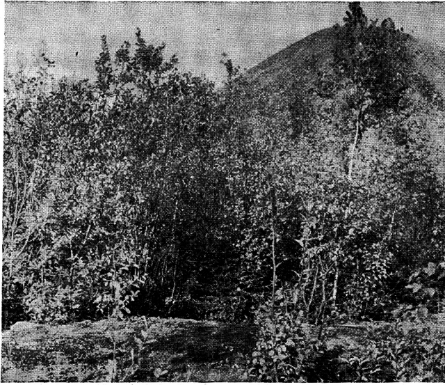
Abb. 7. Granithalde am Filzteich bei Schneeberg. Während die Pionierlaubhölzer ein fast undurchdringliches Dickicht mit Fichten bilden, scheint die Spitzhalde im Hintergrund unbewachsen zu sein. Gneis als Haldengestein.
