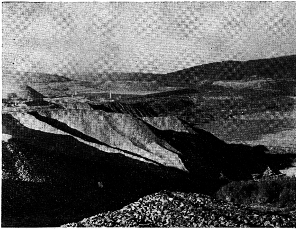
Abb. 1. Johanngeorgenstadt, Blick über die Halden der Erzwäschchen. Der trostlose Charakter der Landschaft wird hauptsächlich durch die Vegetationsarmut der Halden bedingt.
