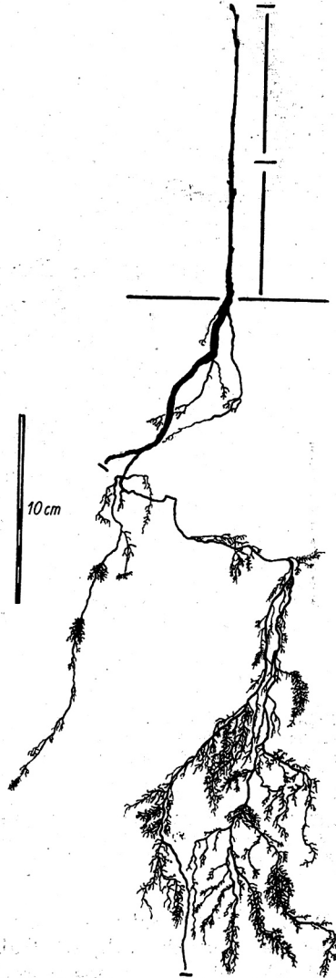
Abb. 5. Wurzelprofil einer zweijährigen Betula pendula vom Plateau einer Wismuthalde in Niederpöbel. Beachtenswert erscheint die besenartige Wurzelauflaufzweigung in Feinbodenklümpchen.
