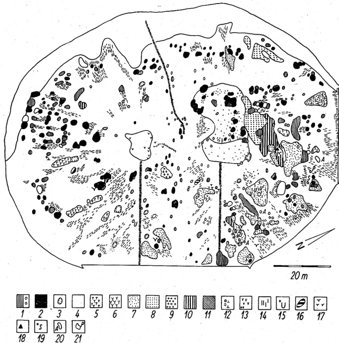
Abb. 13. Wismuthalde in Schneeberg, etwa 300 m westlich vom Rathaus. Sept. 62. Die Schraffen kennzeichnen die Schuttstreifen. An der Westseite der Halde befindet sich an der Basis ein Gebüschsaum mit 70–80 % Deckung. Die Birke überwiegt.
