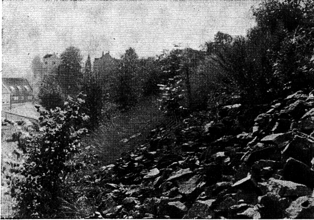
Abb. 11. Terrakonikhalde in Schneeberg. Vegetationsausschnitt vom mittleren Osthang, Blick nach Süden. Im Bild wachsen Tilia platyphyllos , Poa nemoralis , Acer platanoides , Chamaenerion angustifolium , Athyrium filix-femina , Betula pendula .
