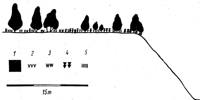
Abb. 15. Wie Abb. 14, Westteil des Haldenkomplexes. Profil SSE-NNW, 2 m breit. Im links anschließenden Haldenteil wachsen noch Aspe, Salweide und Eberesche sowie Ramschia secunda und Epipactis atrorubens in der Feldschicht. 1 Betula pendula , 2 Deschampsia flexuosa — rasig, 3 dgl. — horstig, 4 Cladonia verticillata , 5 Polytrichum piliferum .
