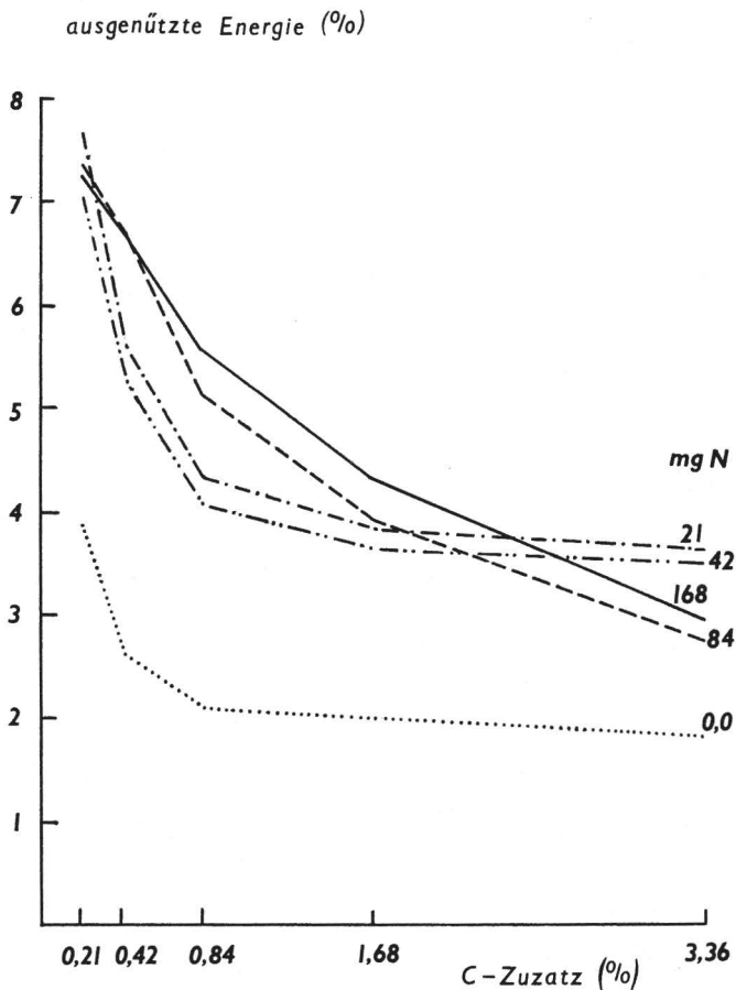
Abb 10. Prozentsatz der freien Energie, die zur Stickstoffimmobilisierung ausgenutzt wird, abhängig von der Strohgabe
